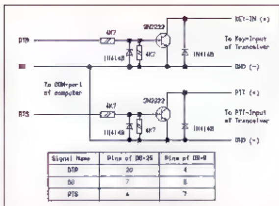
Tekening 1: De interface voor de seriële (COM)-poort.
